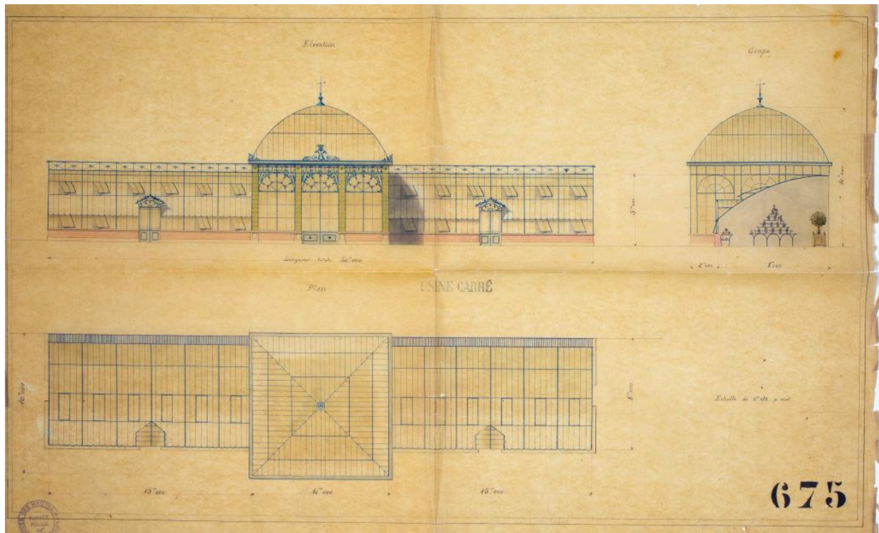
Projet de jardin d'hiver, vue en coupe, plan et en élévation.
