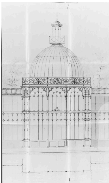
Projet de jardin d'hiver, élévation de la partie centrale. Phot. Philippe Poitou IVR76_20166551172NUCA
