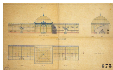
Projet de jardin d'hiver, vue en coupe, plan et en élévation. Phot. Philippe Poitou IVR76_20166551164NUCA
