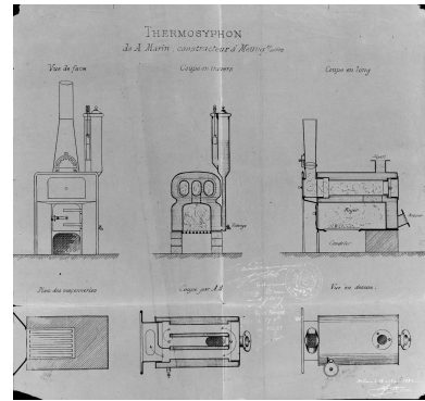
Thermosyphon de A. Marin, dessin. Phot. Philippe Poitou IVR76_20166551183NUCA
