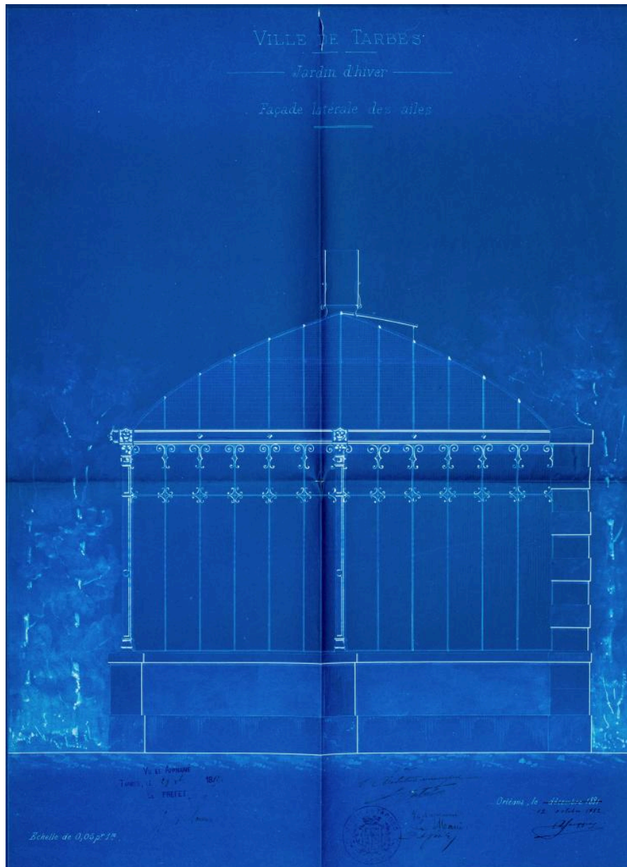
Projet de jardin d'hiver, façade latérale des ailes.
