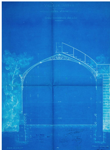
Projet de jardin d'hiver, coupe transversale des ailes. Phot. Philippe Poitou IVR76_20166551177NUCA
