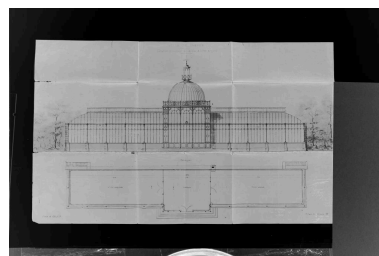
Projet de jardin d'hiver, vue en plan et en élévation, 1881. Phot. Philippe Poitou IVR76_20166551168NUCA
