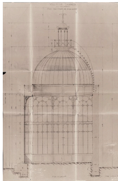
Projet de jardin d'hiver, coupe transversale du dôme central. Phot. Philippe Poitou IVR76_20166551170NUCA
