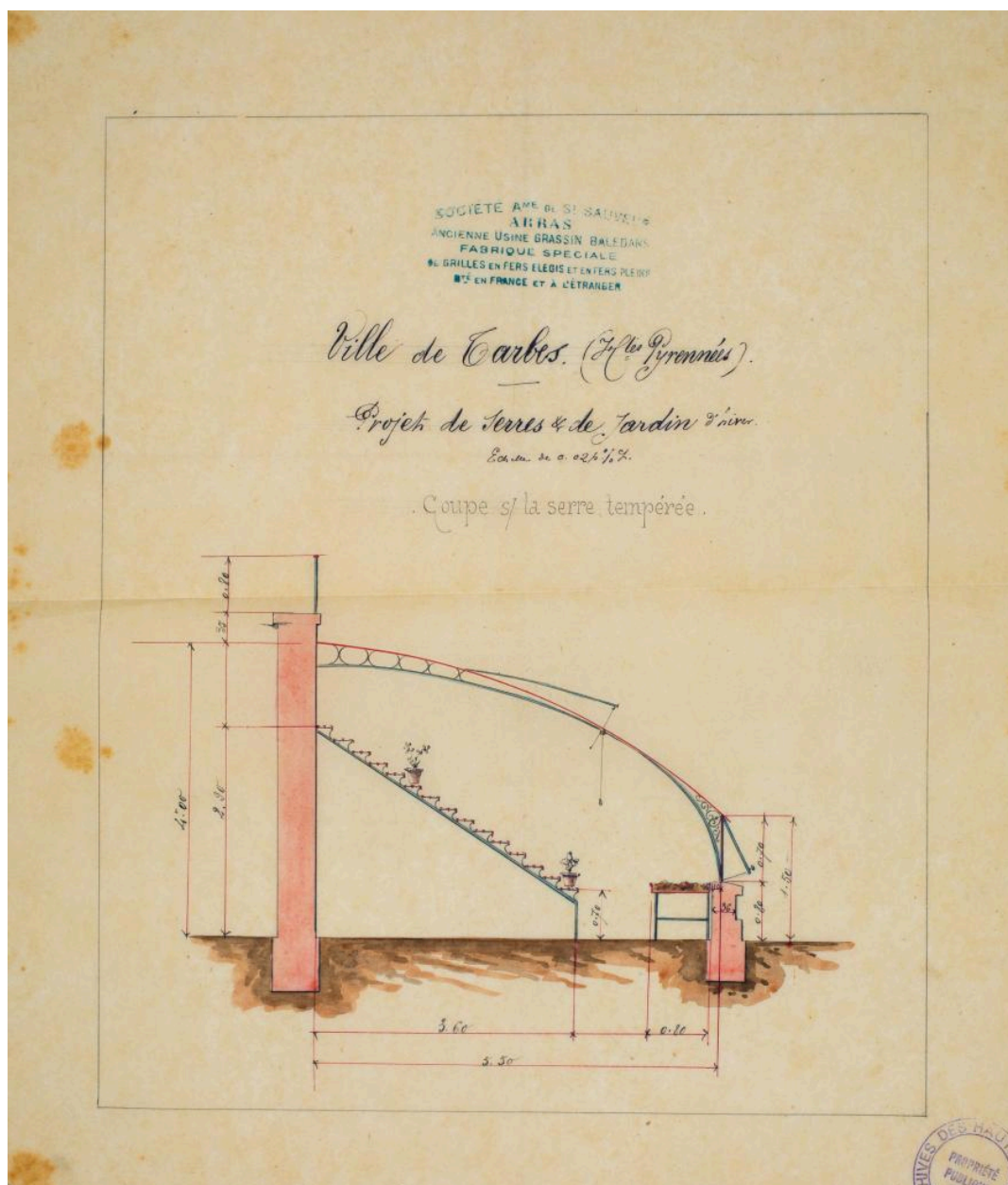
Projet de serres et de jardin d'hiver par la société de Saint-Sauveur, Arras, 1881.
