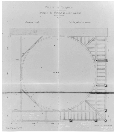
Jardin d'hiver, détail du plafond du dôme central. Phot. Philippe Poitou IVR76_20166551176NUCA
