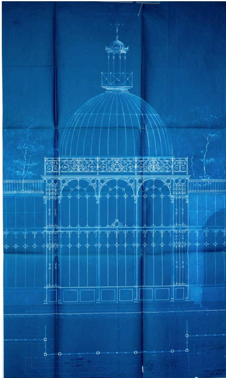
Projet de jardin d'hiver, élévation de la partie centrale.
