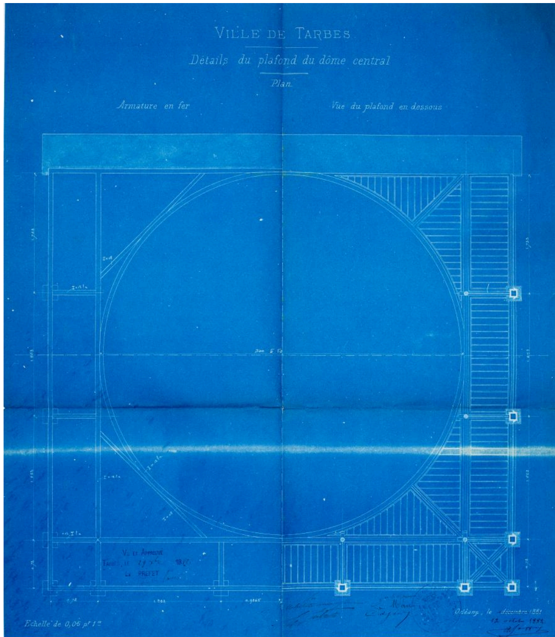
Jardin d'hiver, détail du plafond du dôme central.
