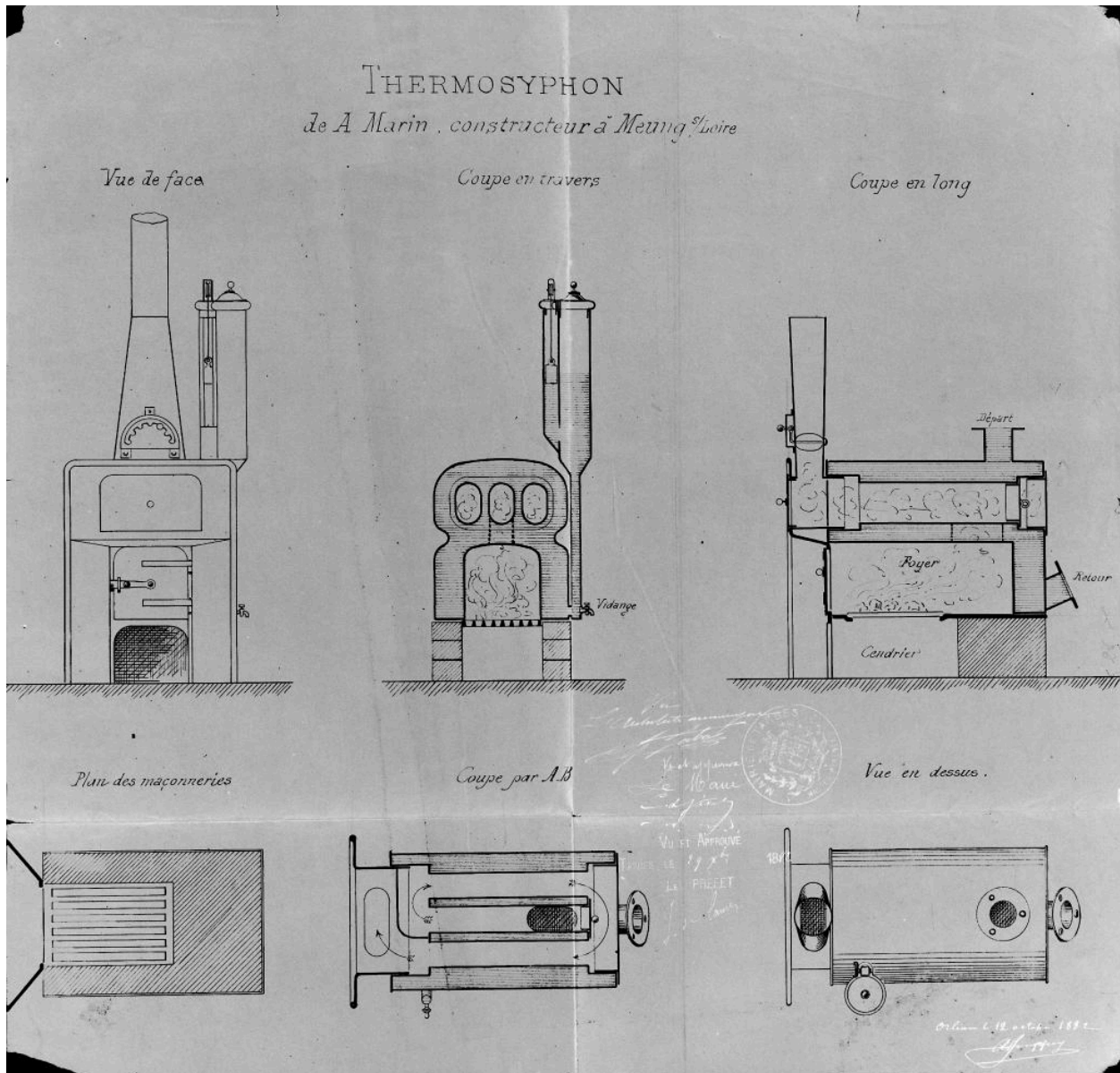
Thermosiphon de A. Marin, dessin.
