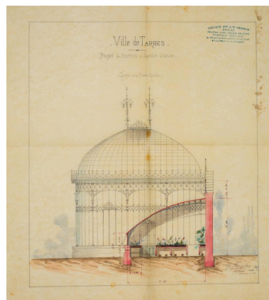
Projet de serres et de jardin d'hiver par la société de Saint-Sauveur, Arras, 1881. Phot. Philippe Poitou IVR76_20166551162NUCA
