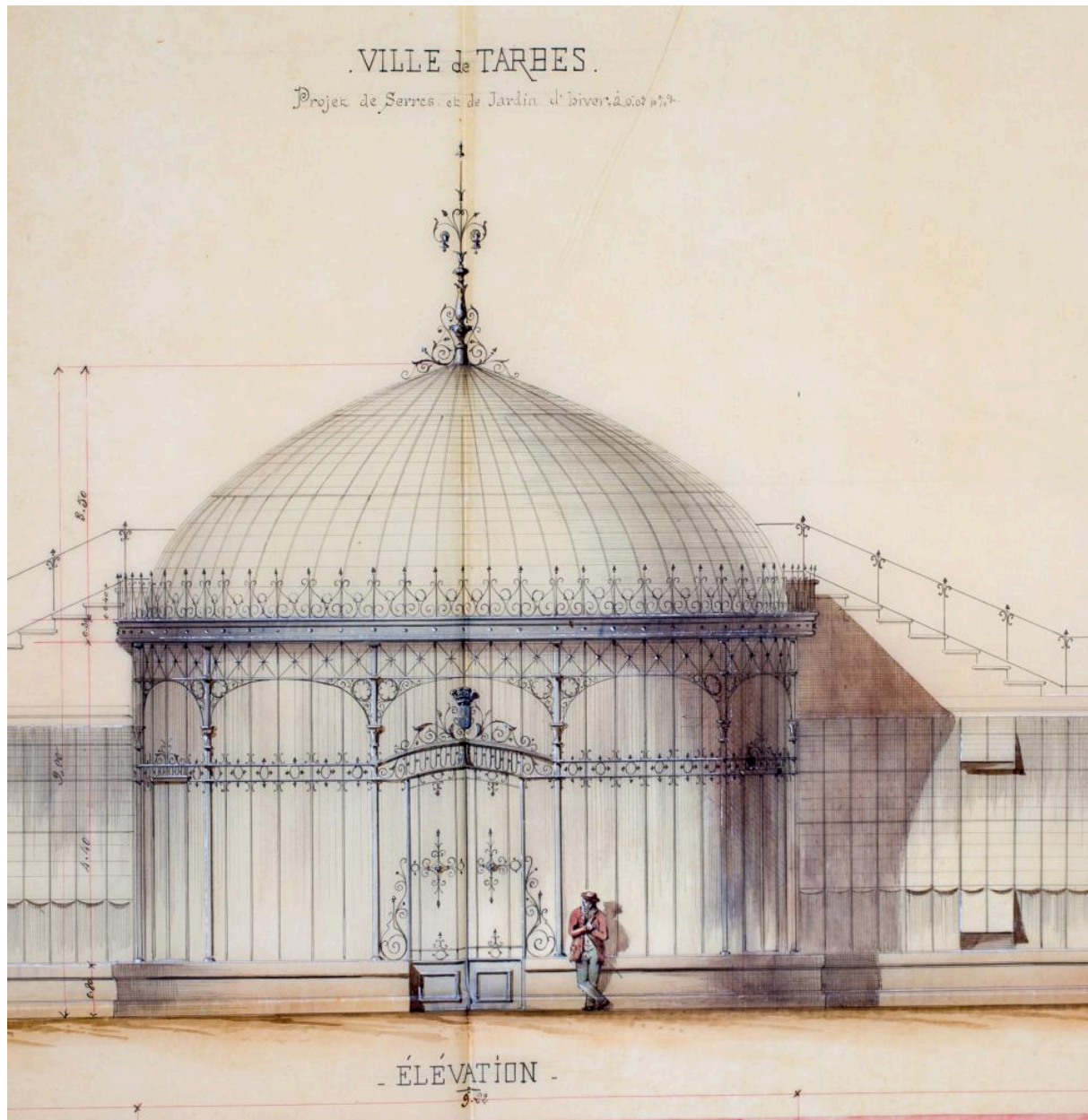
Projet de serres et de jardin d'hiver par la société de Saint-Sauveur, Arras, 1881 (élévation).
