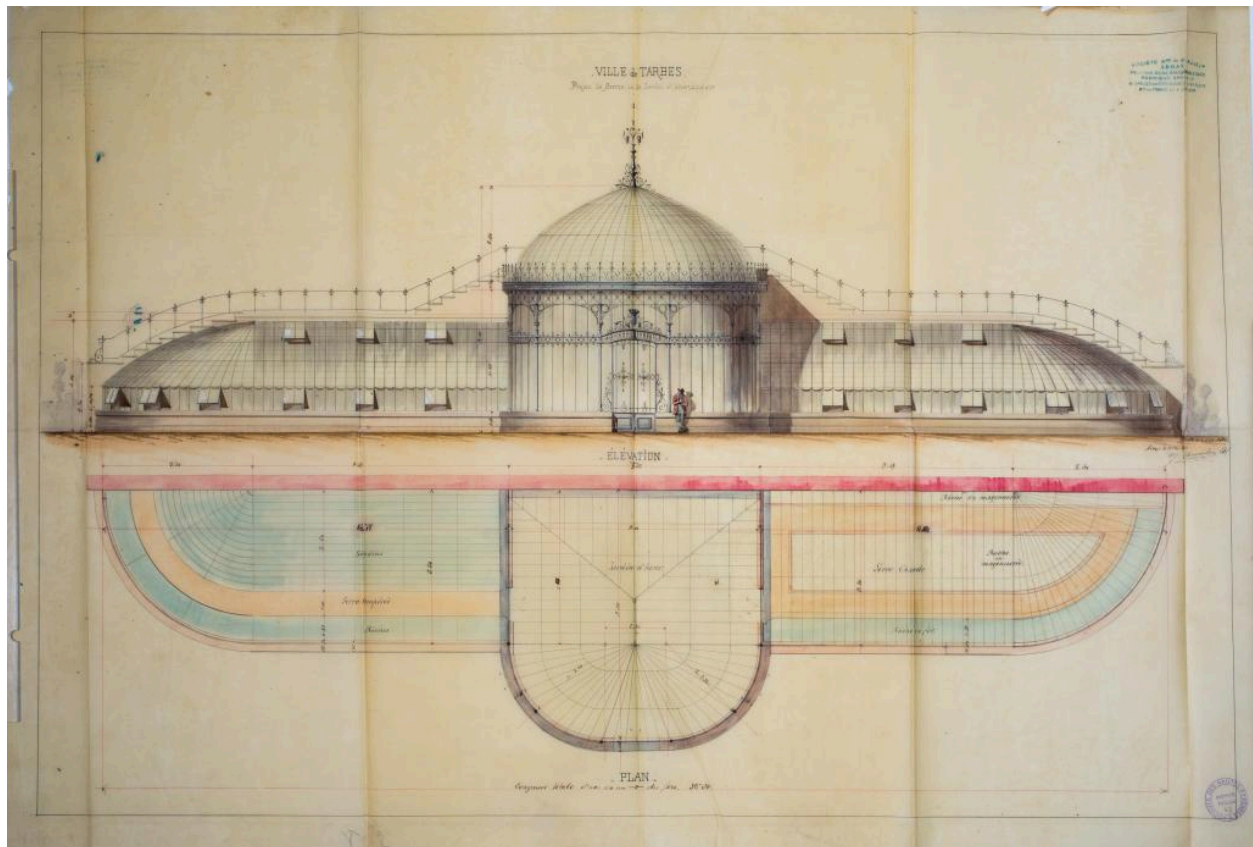
Projet de serres et de jardin d'hiver par la société de Saint-Sauveur, Arras, 1881.
