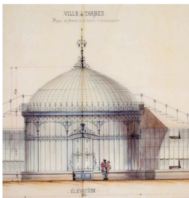
Projet de serres et de jardin d'hiver par la société de Saint-Sauveur, Arras, 1881 (élévation). Phot. Philippe Poitou IVR76_20166551159NUCA
