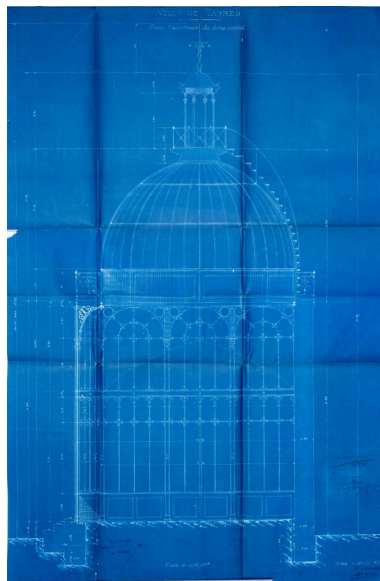
Projet de jardin d'hiver, coupe transversale du dôme central. Phot. Philippe Poitou IVR76_20166551169NUCA
