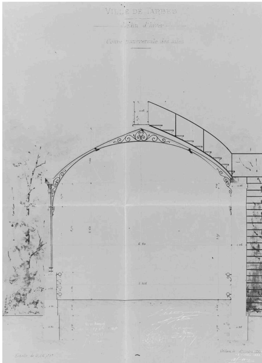
Projet de jardin d'hiver, coupe transversale des ailes.
