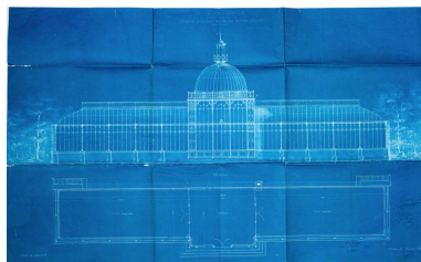
Projet de jardin d'hiver, vue en plan et en élévation, 1881. Phot. Philippe Poitou IVR76_20166551167NUCA
