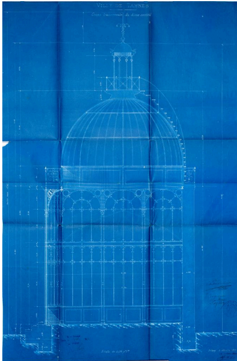
Projet de jardin d'hiver, coupe transversale du dôme central.
