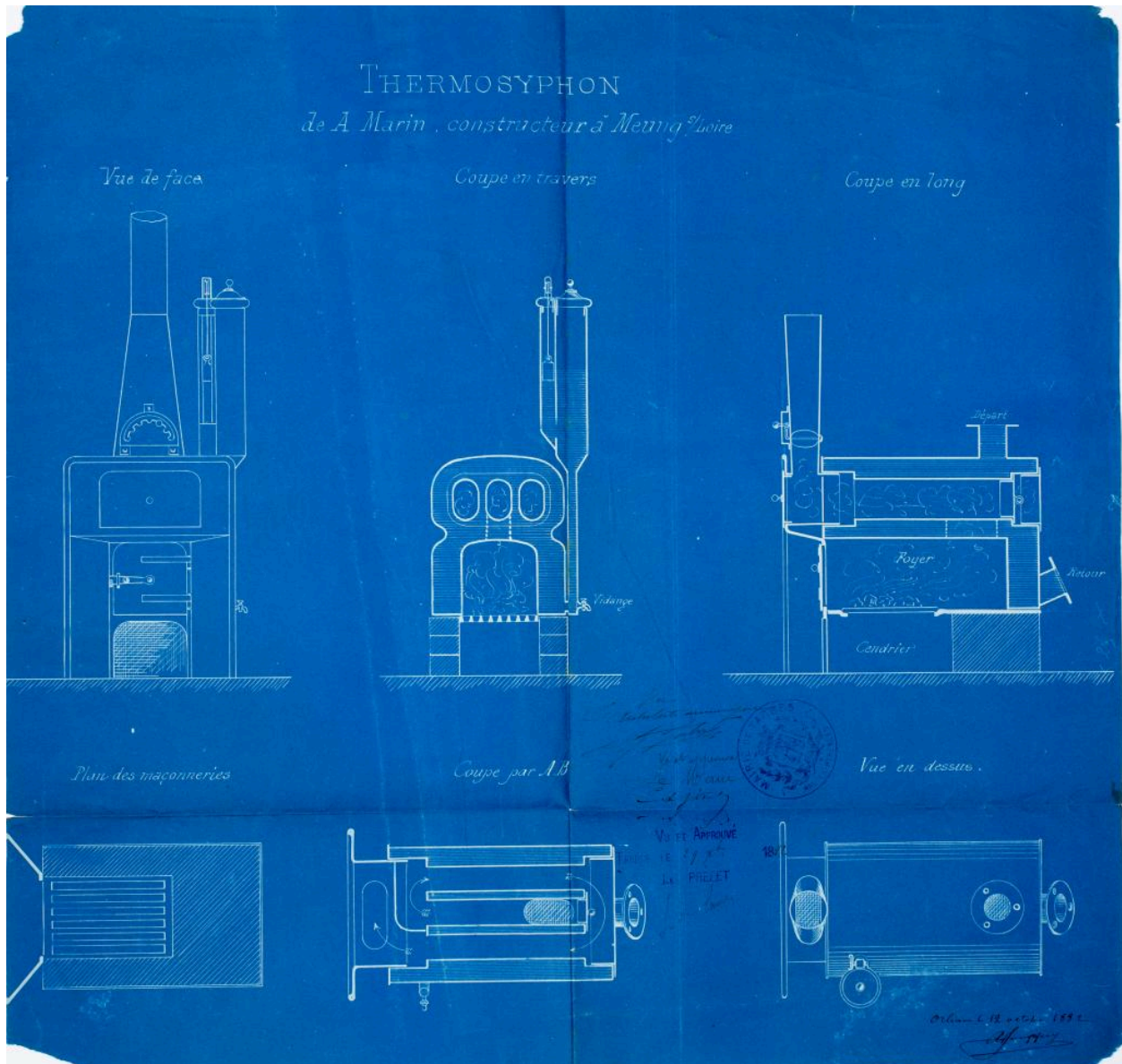
Thermosiphon de A. Marin, calque bleu.
