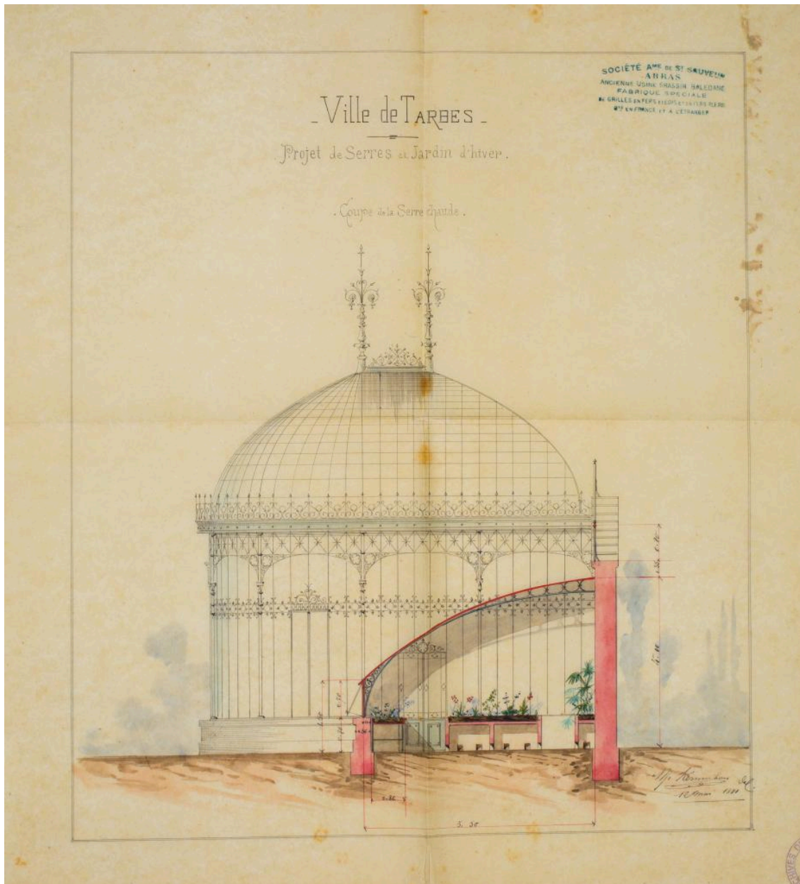
Projet de serres et de jardin d'hiver par la société de Saint-Sauveur, Arras, 1881.
