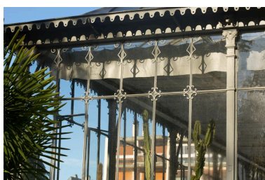
Profilé de l'armature métallique de la serre : détail. Phot. Philippe Poitou IVR73_20156551078NUCA
