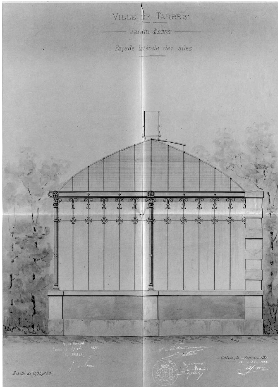
Projet de jardin d'hiver, élévation latérale, 1881.
