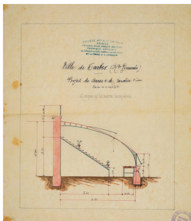
Projet de serres et de jardin d'hiver par la société de Saint-Sauveur, Arras, 1881. Phot. Philippe Poitou IVR76_20166551163NUCA
