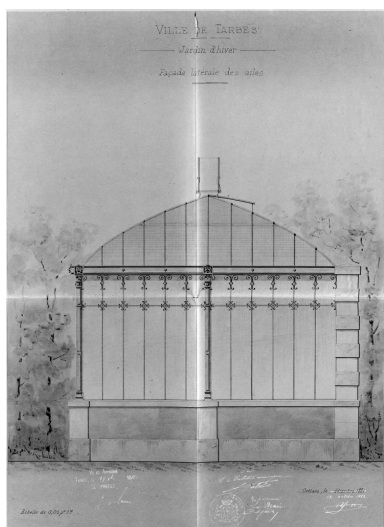
Projet de jardin d'hiver, élévation latérale, 1881. Phot. Philippe Poitou IVR76_20166551181NUCA
