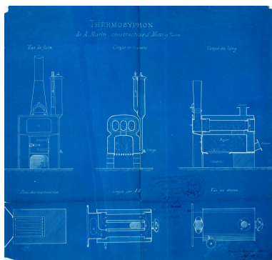
Thermosyphon de A. Marin, calque bleu. Phot. Philippe Poitou IVR76_20166551182NUCA
